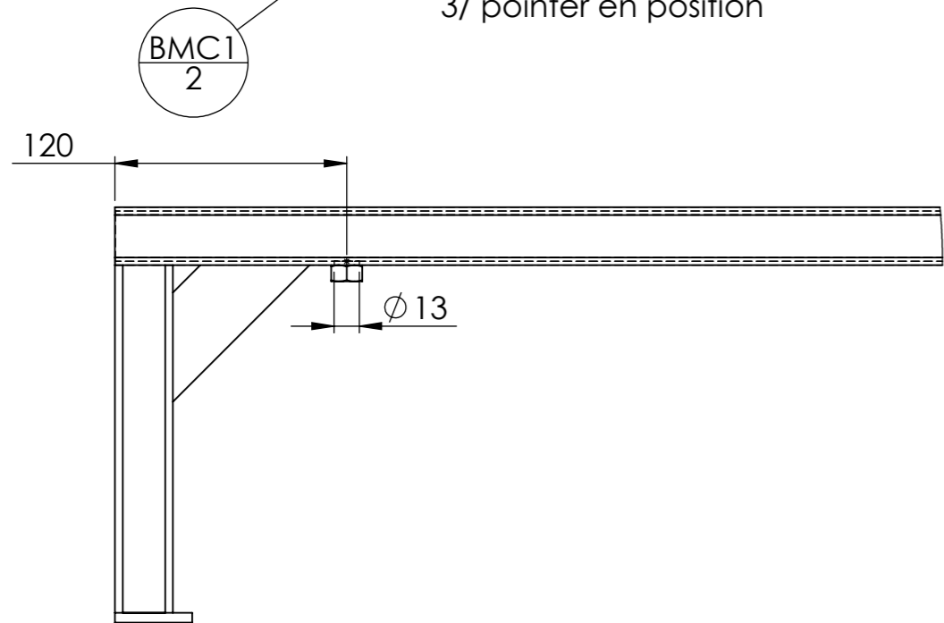
DÉTAIL A ECHELLE 2 : 7
