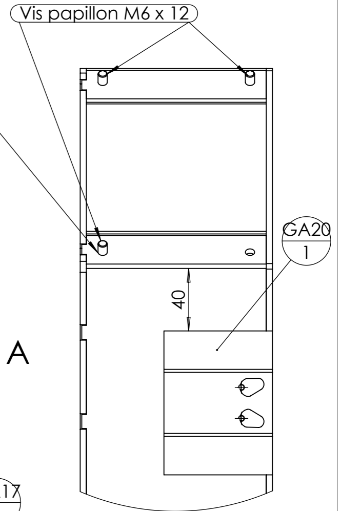
DÉTAIL A ECHELLE 2 : 5
