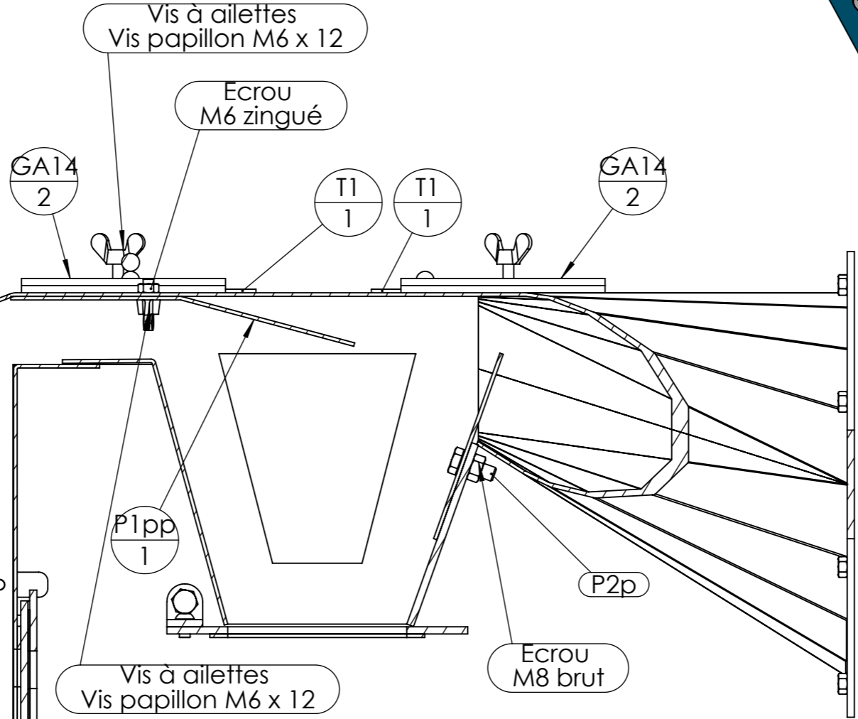
COUPE S-S ECHELLE 1 : 3
