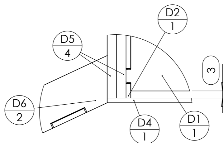
DÉTAIL A ECHELLE 1 : 1
