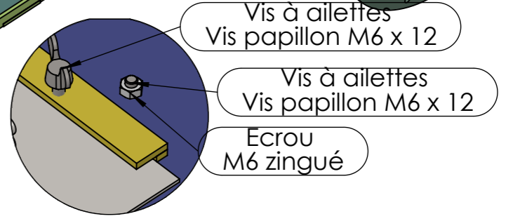
DÉTAIL T ECHELLE 2 : 5
