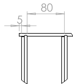
DÉTAIL O ECHELLE 1 : 5
