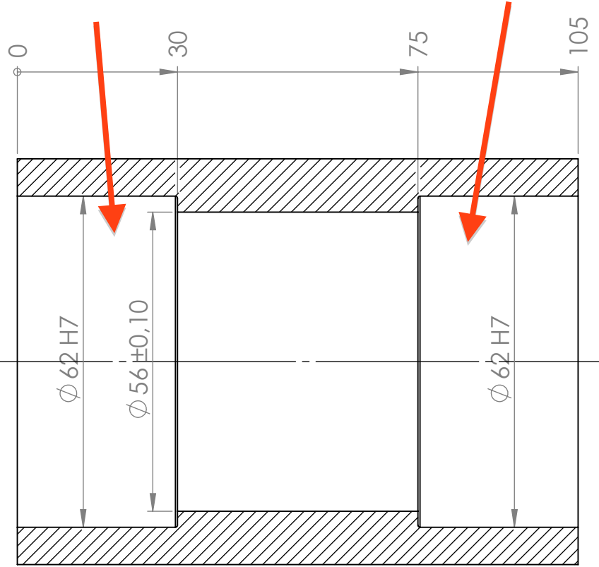
COUPE C-C
