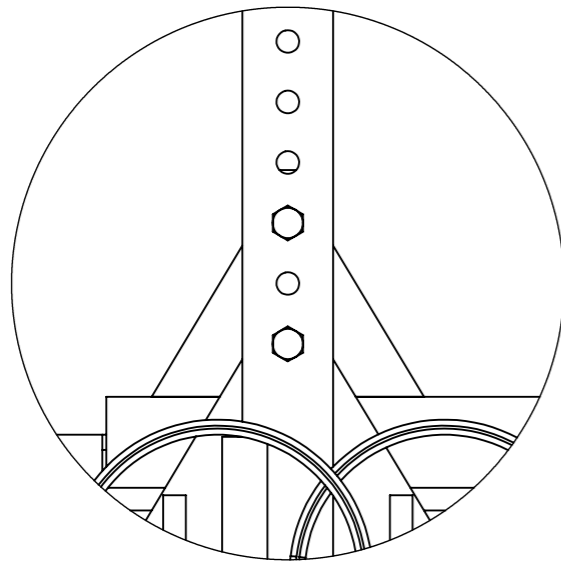
DÉTAIL B ECHELLE 1 : 5
